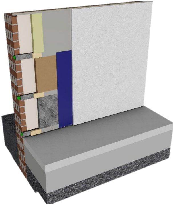
No Battens
